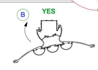
Agganciare la lampada di lato per collegare il cavo di alimentazione
